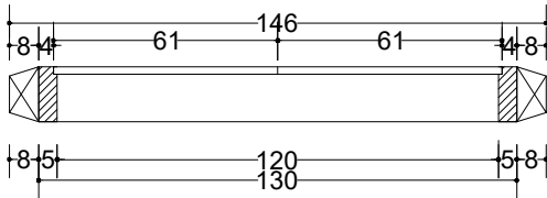
P1 (1 BUAH) SKALA 1:20
