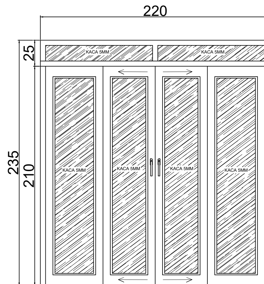
PJ2 (1 BUAH) SKALA 1:20
