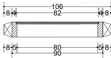
P3 (1 BUAH) SKALA 1:20
