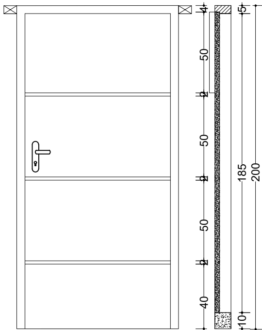
P3 (1 BUAH) SKALA 1:20
