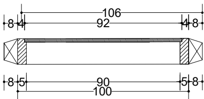
P2 (6 BUAH) SKALA 1:20
